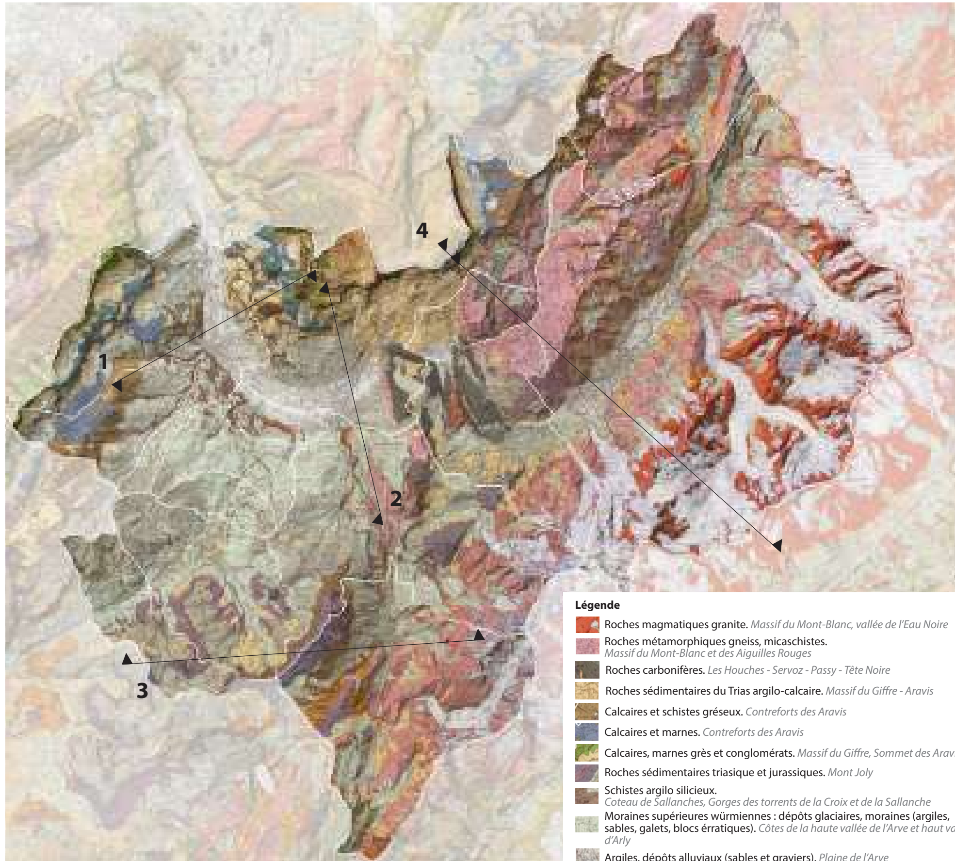
CARTOGRAPHIE DE LA GÉOLOGIE DU SOCLE
